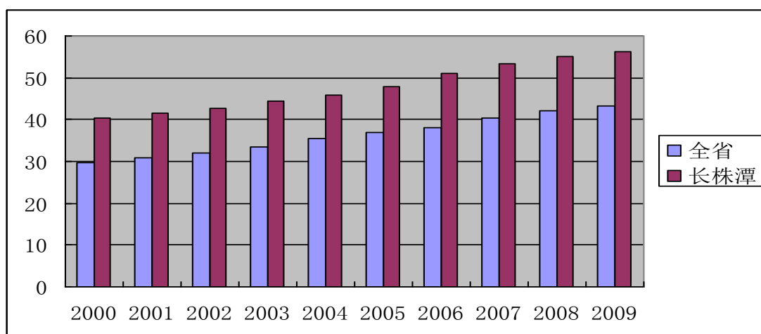
图 3-3: 长株潭城市化水平 (单位: %)
