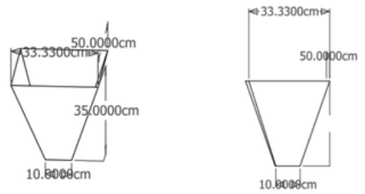
Fig. 7. Cone Dimensions
