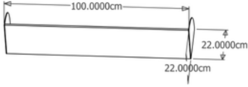
Fig. 9. Hopper Lid Dimensions
