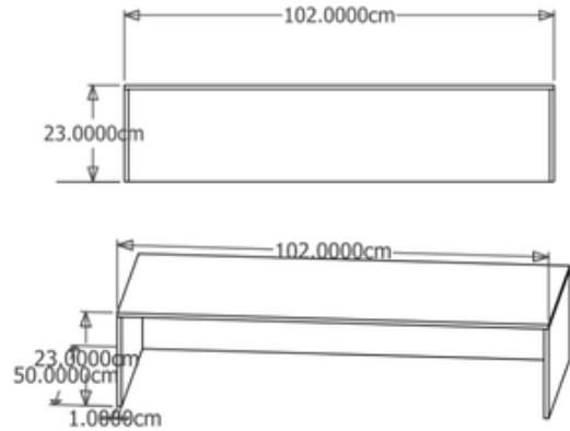
Fig. 8. Box Dimensions
