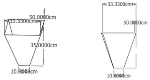
Fig. 7. Cone Dimensions
