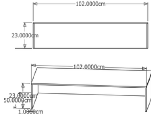
Fig. 8. Box Dimensions
