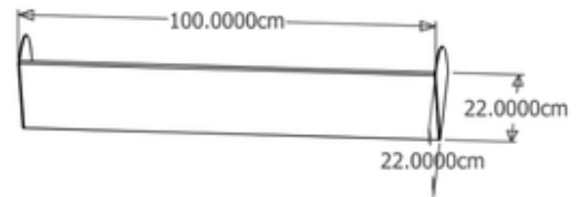
Fig. 9. Hopper Lid Dimensions
