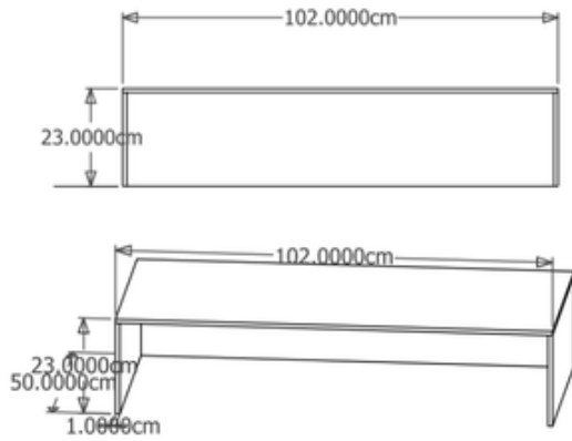
Fig. 8. Box Dimensions
