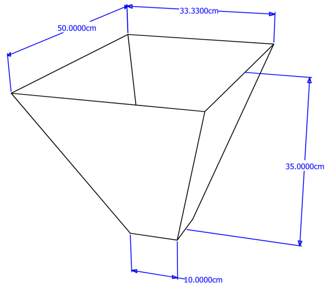
Hopper Dimensions
