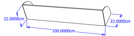
Fig. 9. Hopper Lid Dimensions
