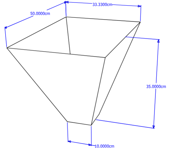
Fig. 7. Cone Dimensions
