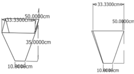
Fig. 7. Cone Dimensions
