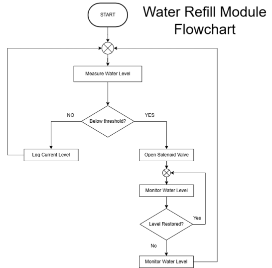
Fig. 14. Water Refill Module Flowchart
