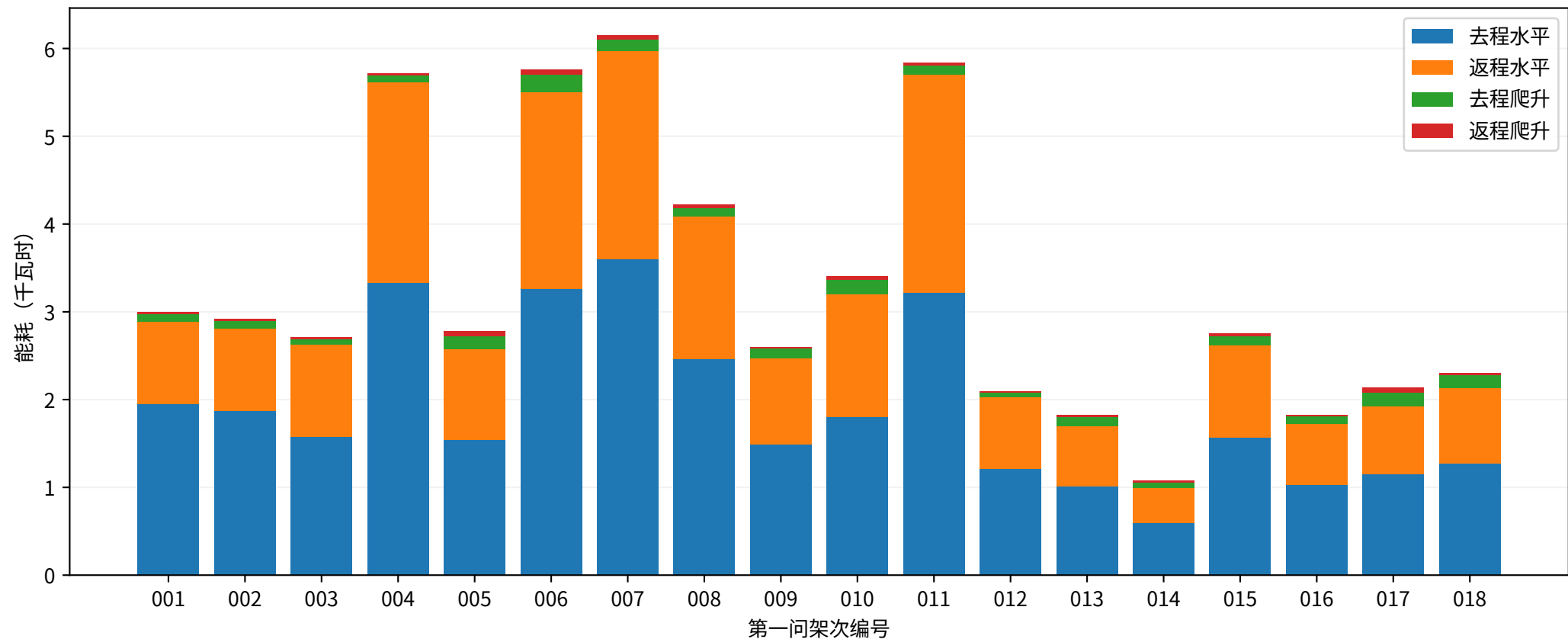
第一问：逐架次往返能耗分解
