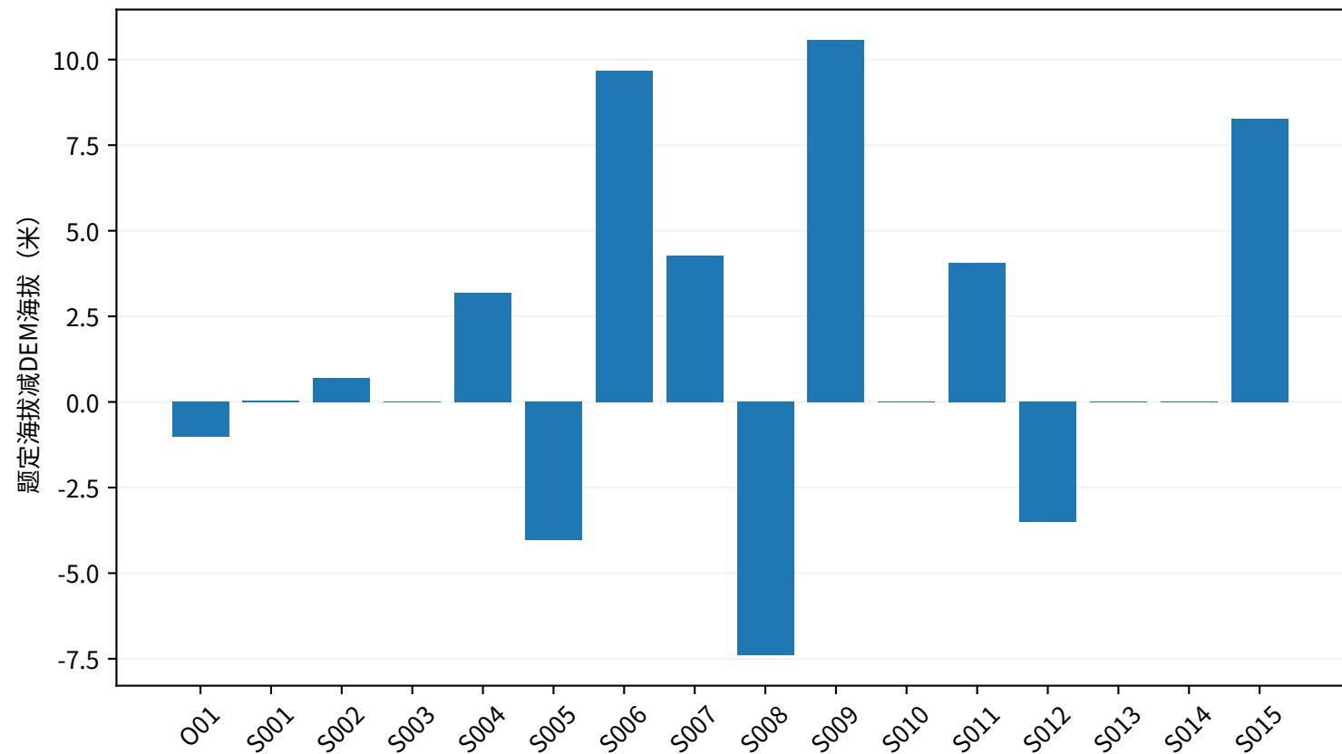
数据核查：题定节点海拔与DEM像元差异
