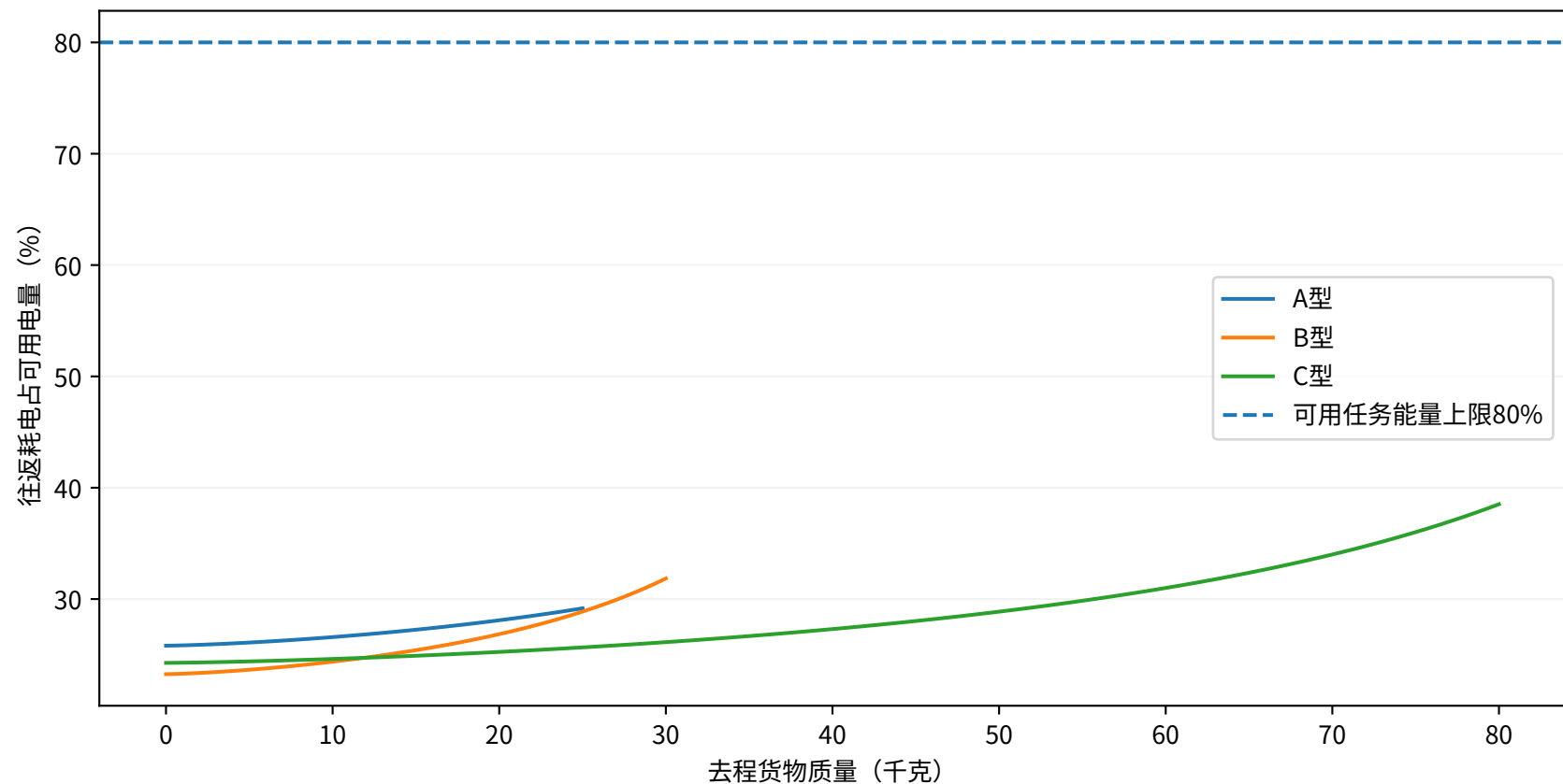
第一问：S001载荷—能量可行边界
