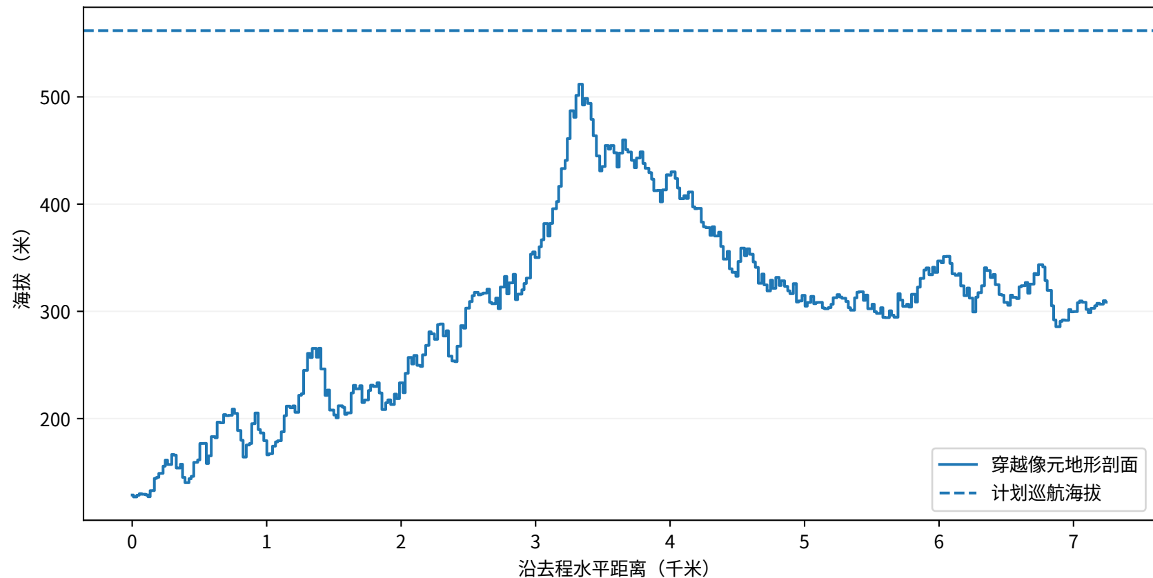
第一问：O01至S003沿线地形与净空
