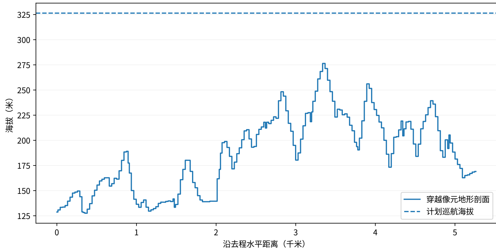
第一问：001至S005沿线地形与净空
