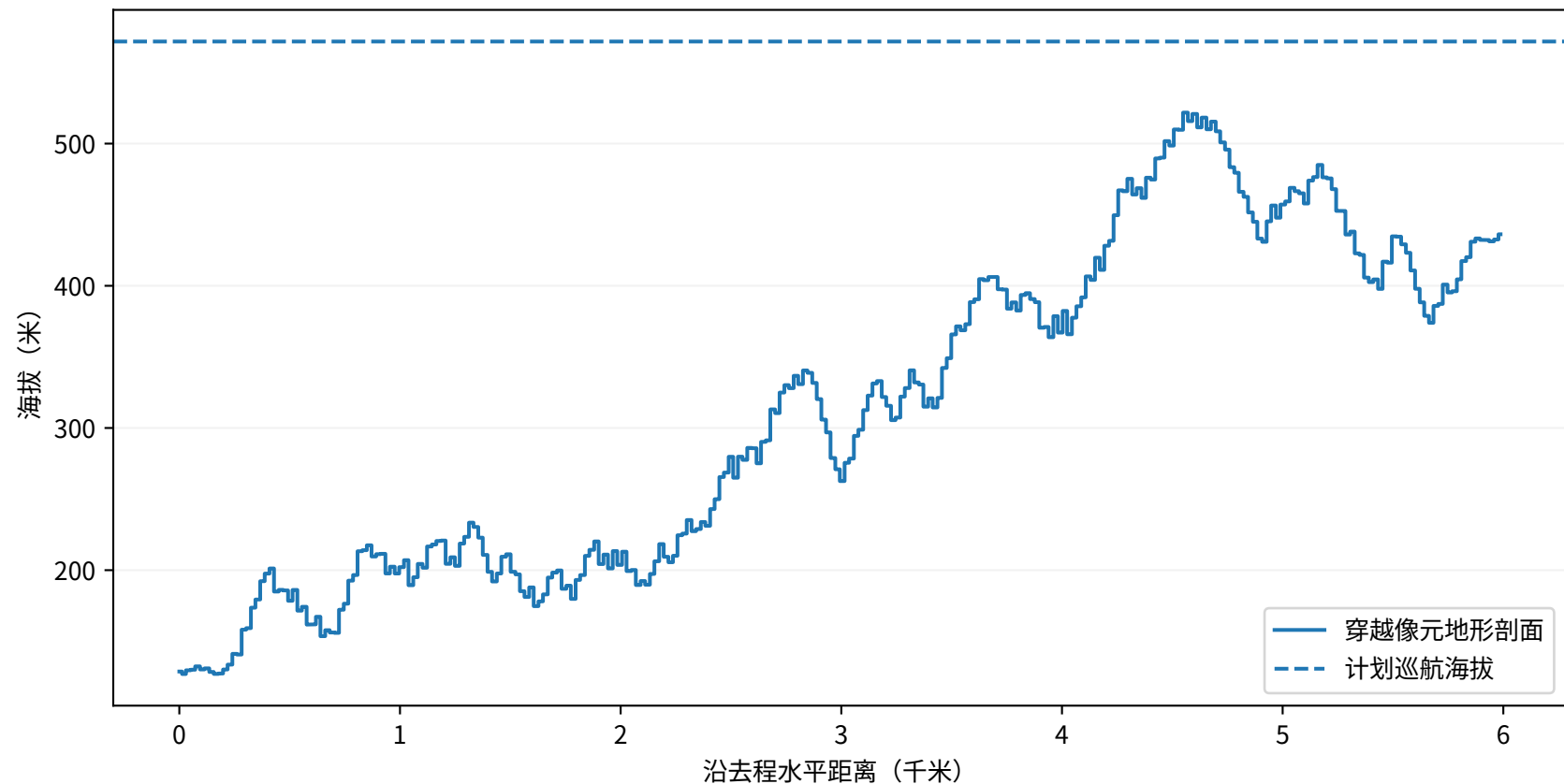
第一问：O01至S015沿线地形与净空
