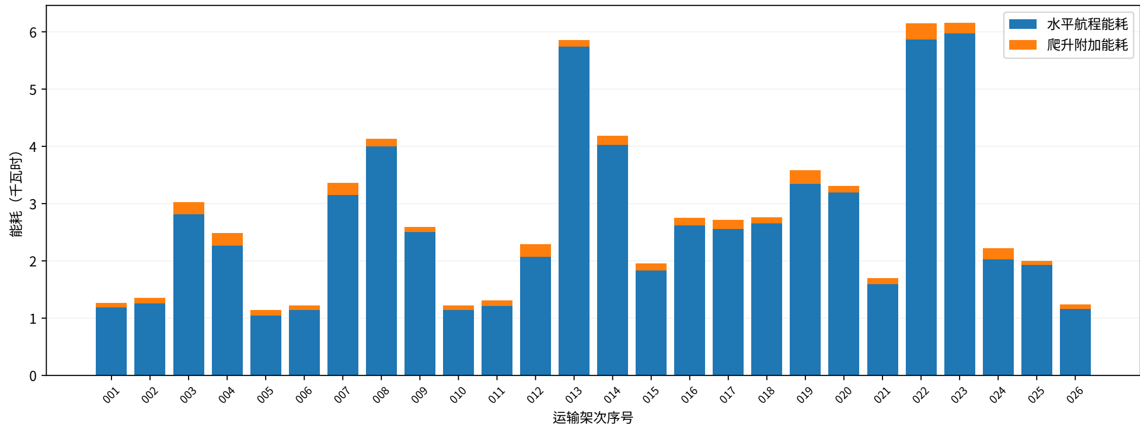
Q2：逐航段汇总的运输能耗分项
