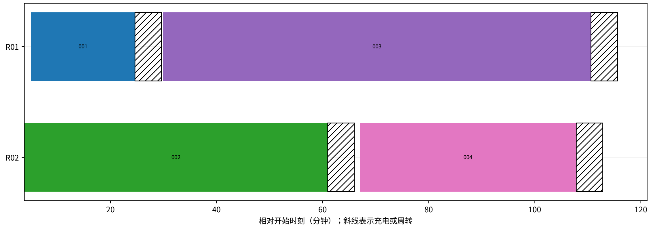
第三问：中继无人机任务及周转
