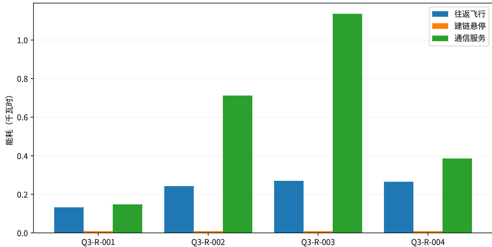
第三问：每次中继任务能耗组成
