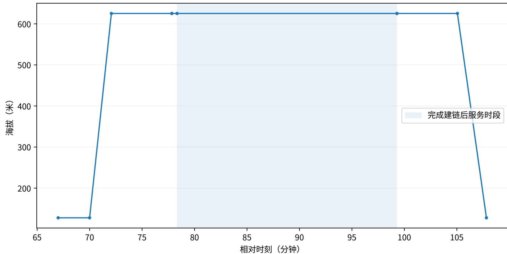
第三问：Q3-R-004完整飞行及服务剖面
