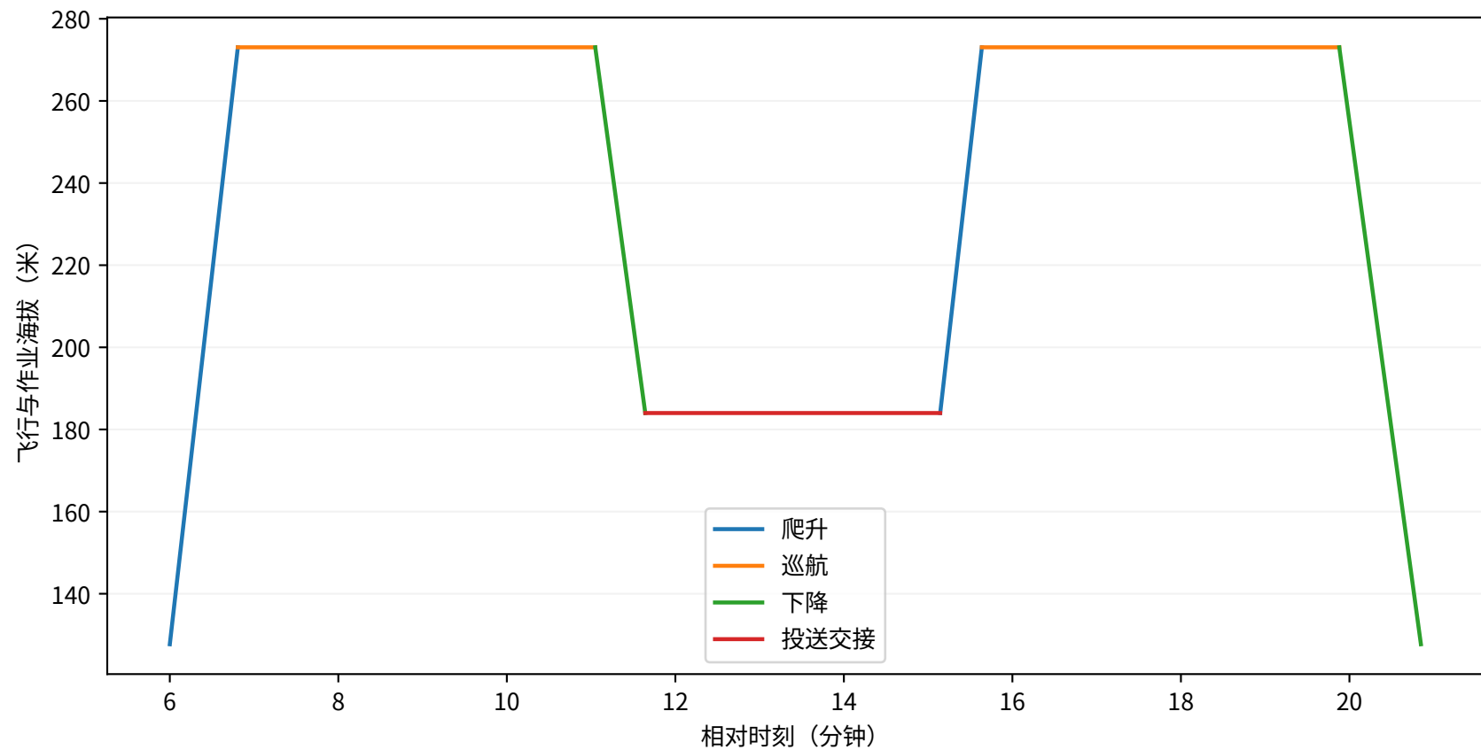
第三问：Q3-T-002逐阶段高度剖面
