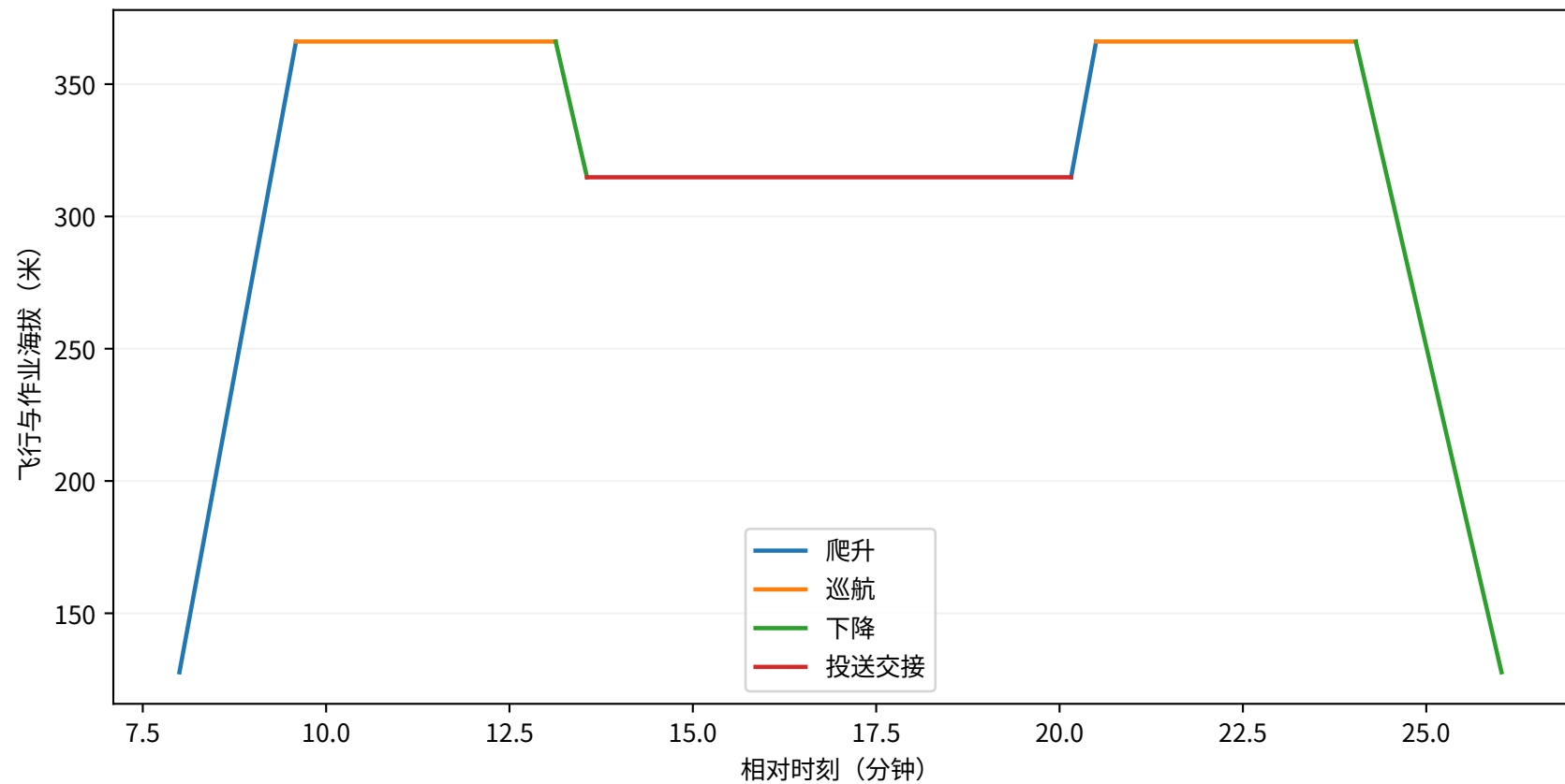
第三问：Q3-T-007逐阶段高度剖面
