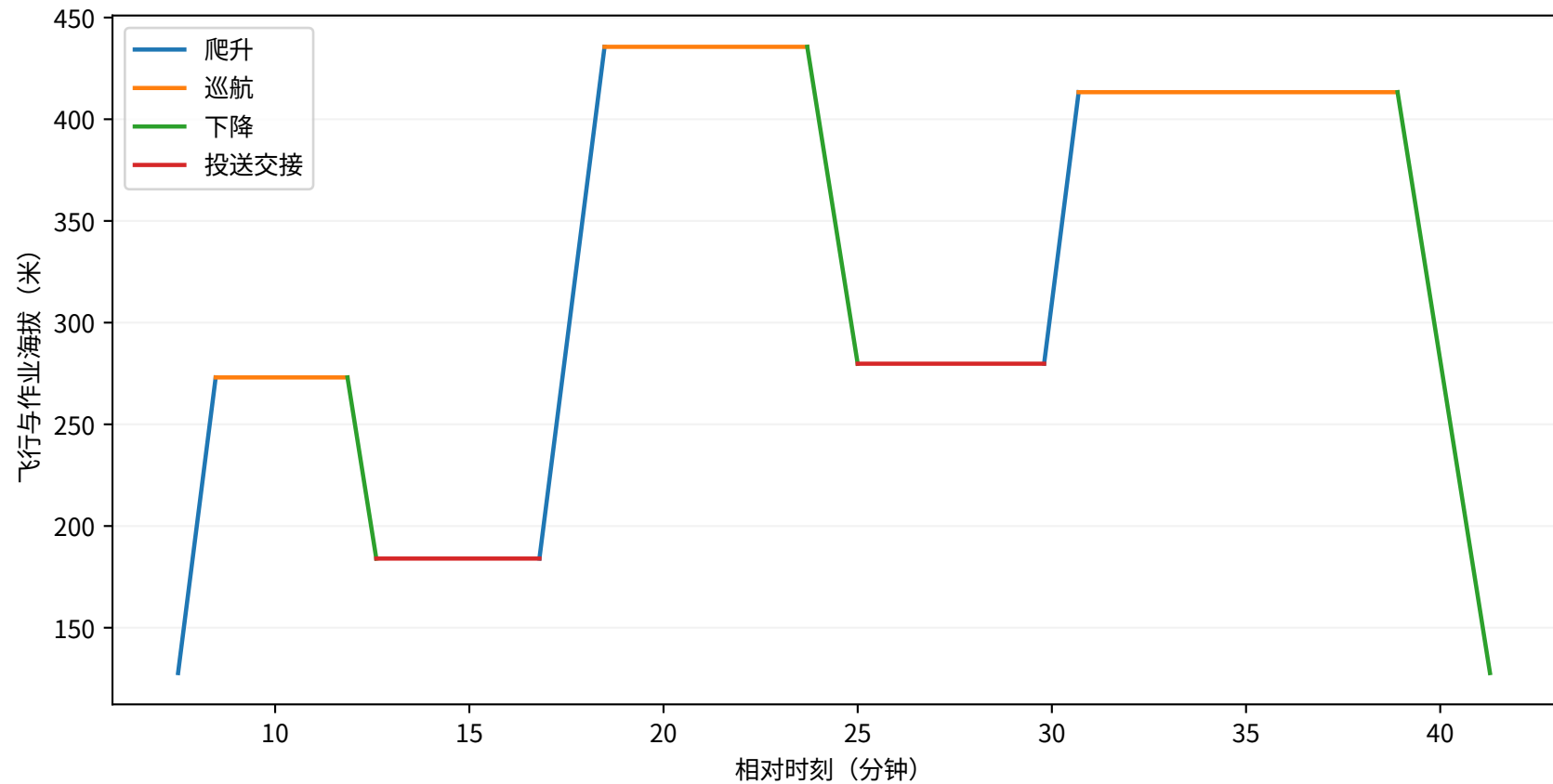
第三问：Q3-T-008逐阶段高度剖面
