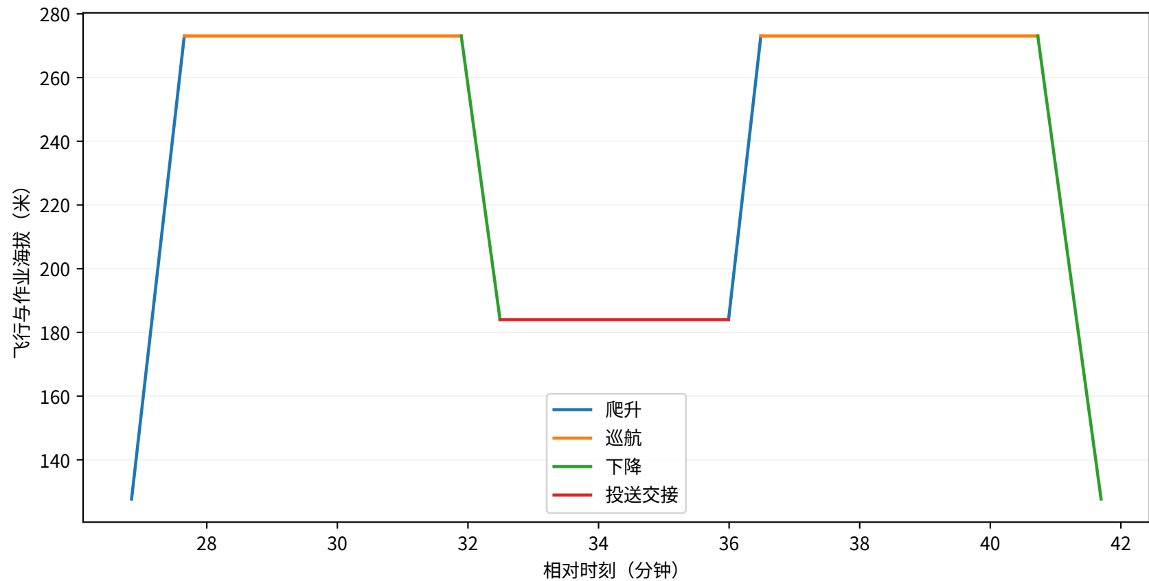
第三问：Q3-T-009逐阶段高度剖面
