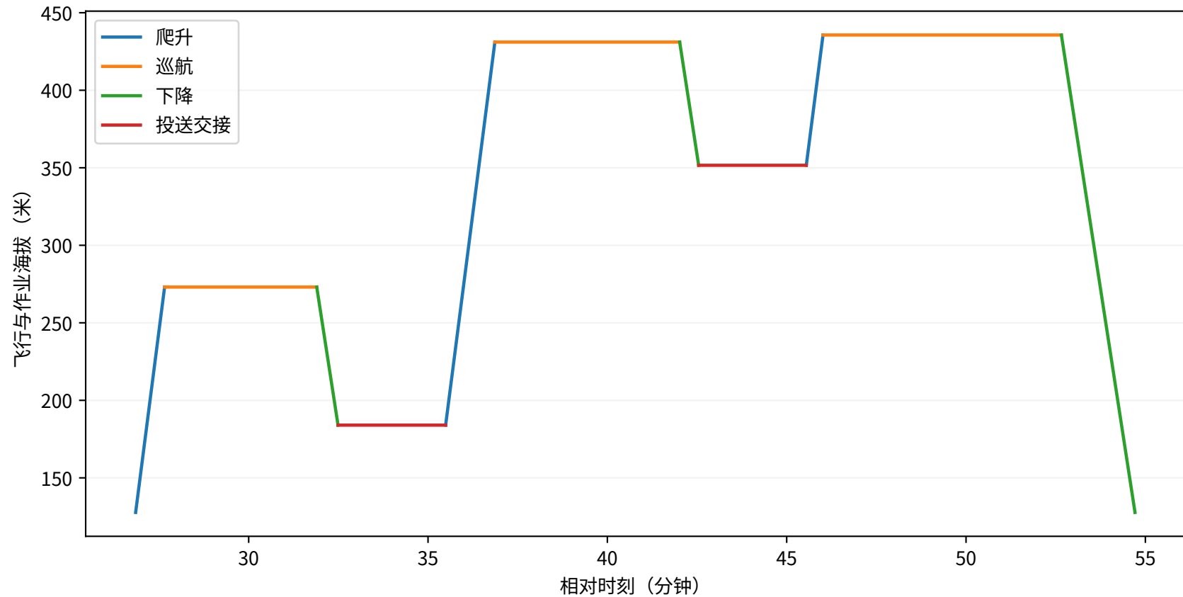
第三问：Q3-T-010逐阶段高度剖面
