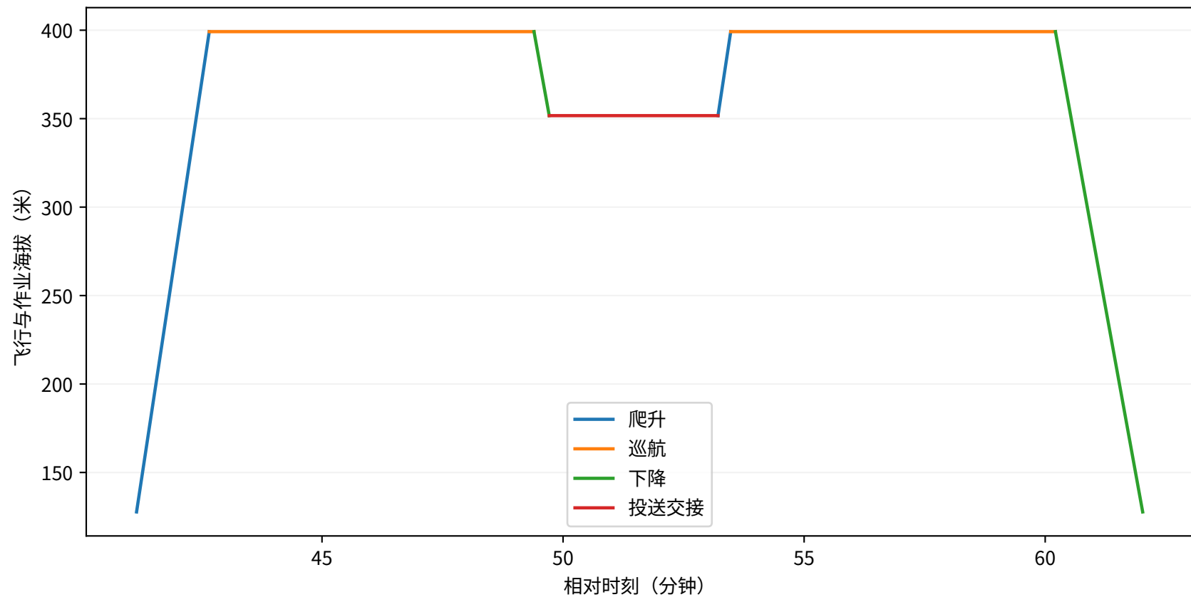
第三问：Q3-T-014逐阶段高度剖面
