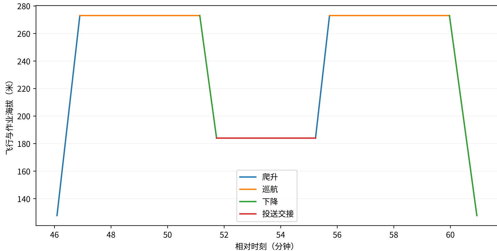
第三问：Q3-T-015逐阶段高度剖面
