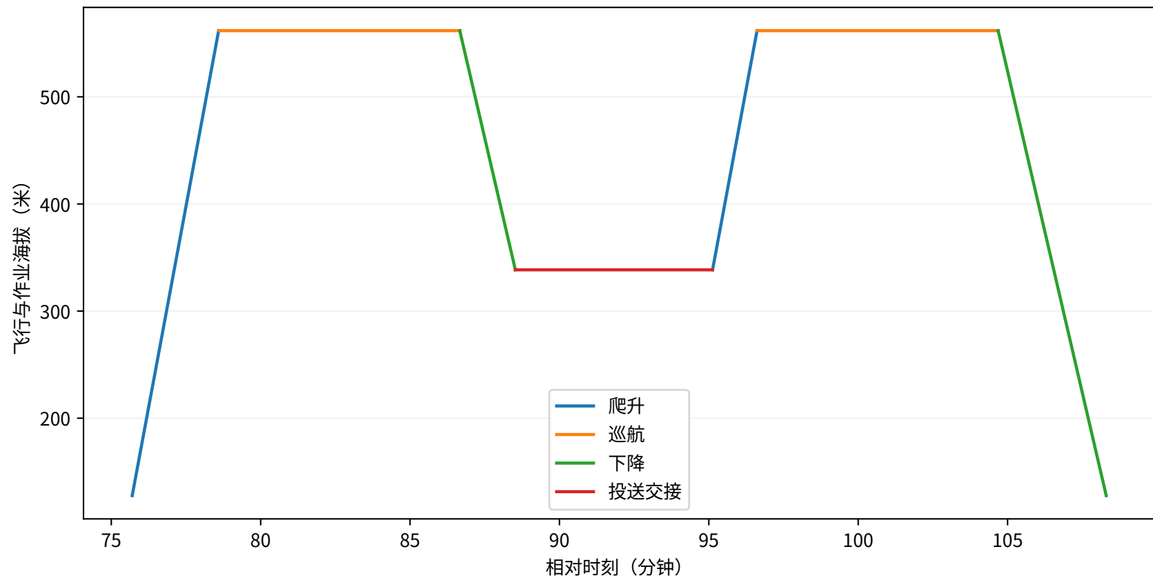
第三问：Q3-T-022逐阶段高度剖面
