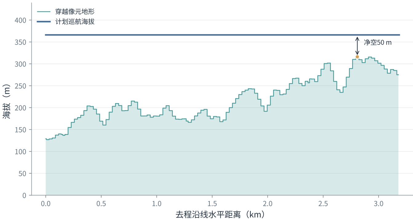
第一问：O01至S006沿线地形与净空
