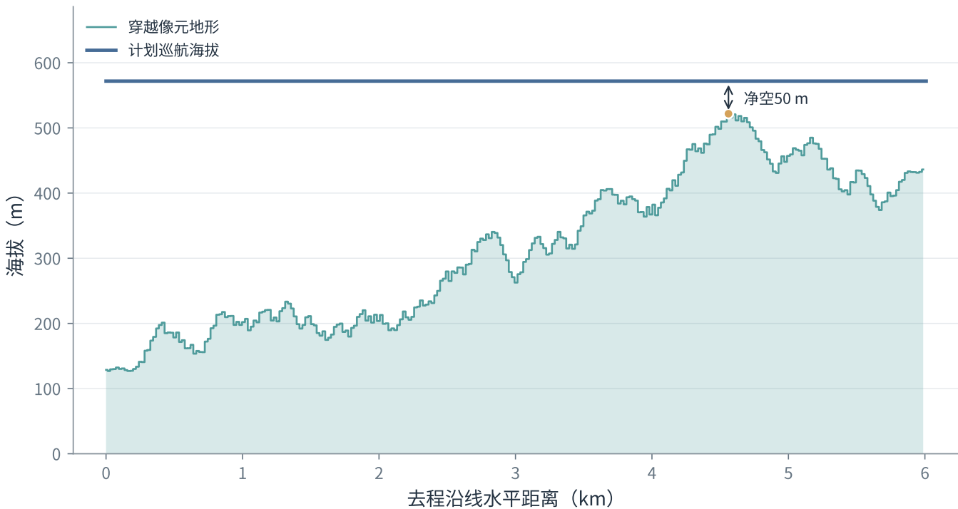
第一问：001至S015沿线地形与净空
