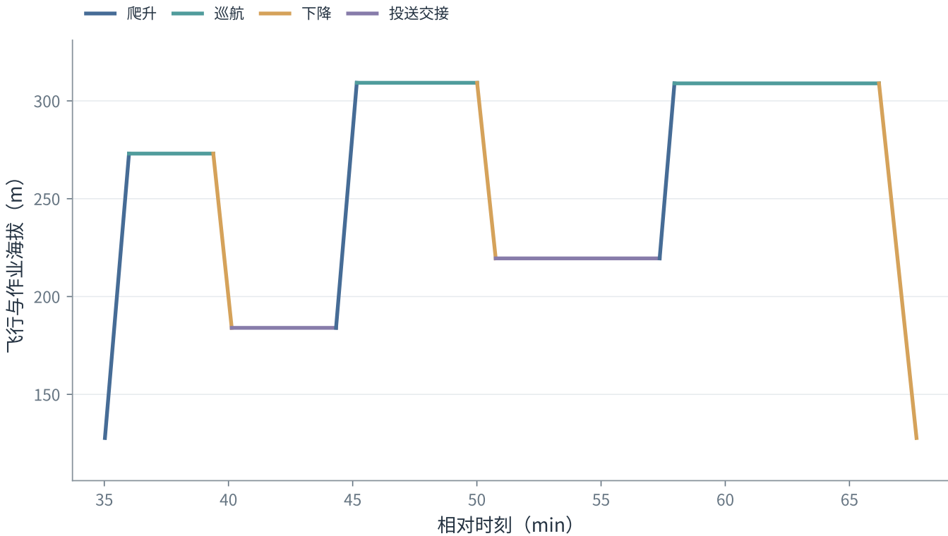
第三问：Q3-T-011逐阶段高度剖面
