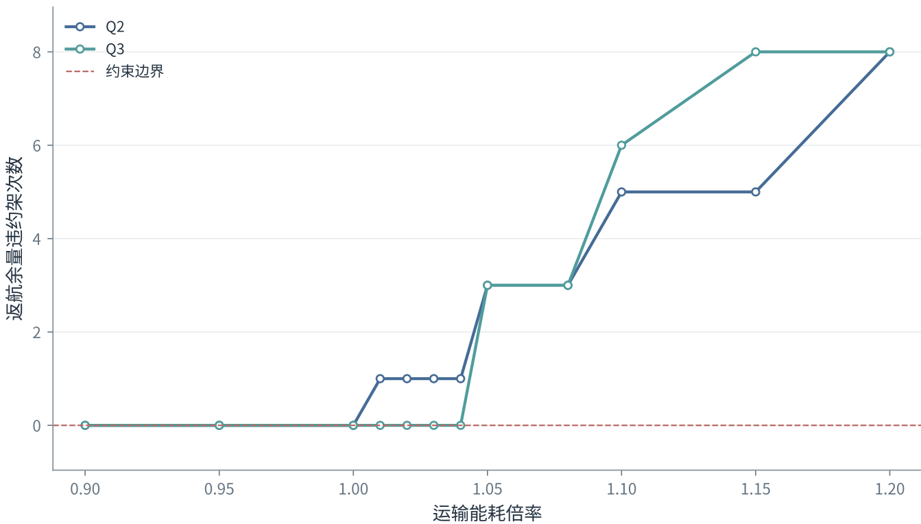
闭环压力测试：运输能耗扰动导致的安全余量违约
