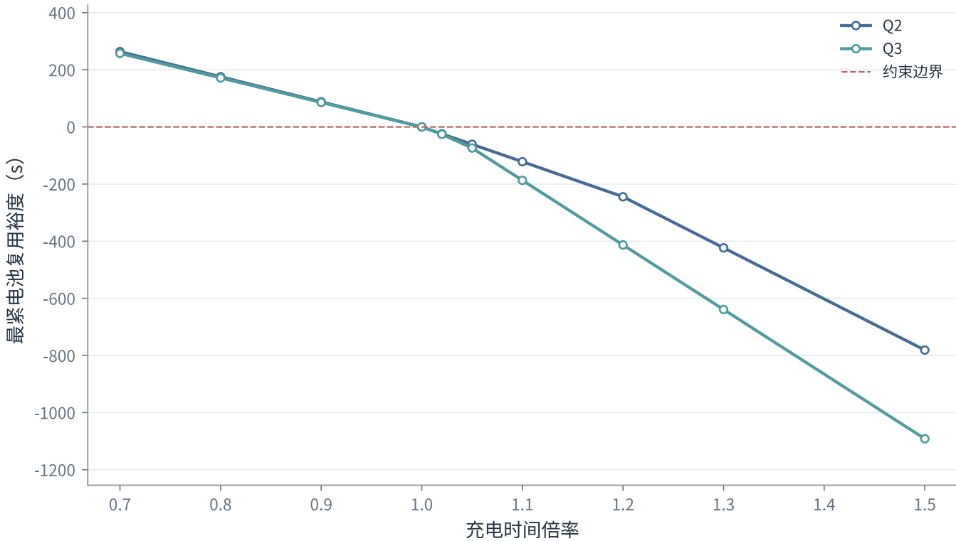
闭环压力测试：充电时间扰动与下一次任务准备裕度
