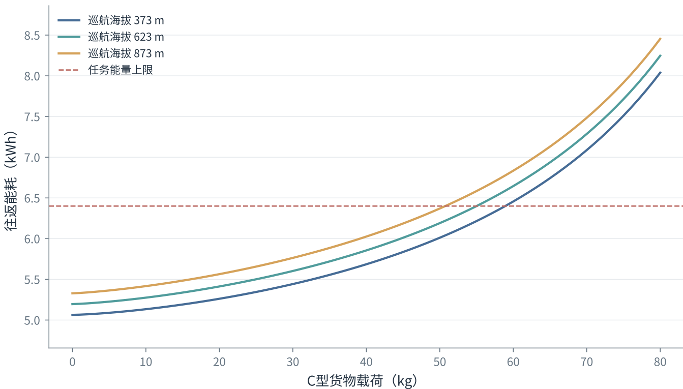
巡航海拔改变时的载荷—能耗截面
