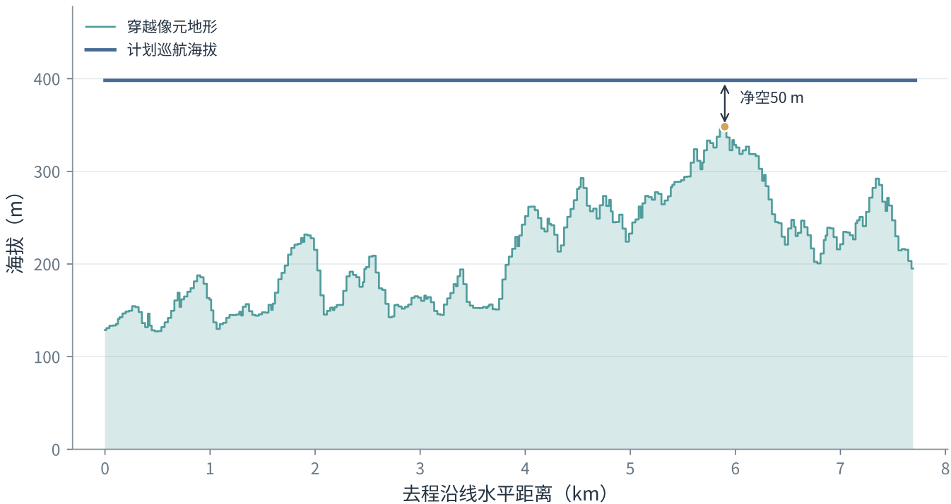
第一问：O01至S004沿线地形与净空
