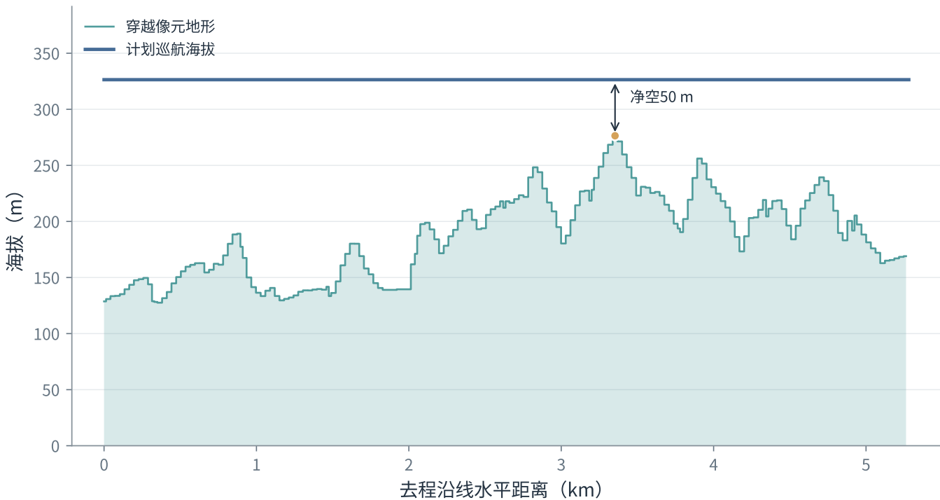
第一问：O01至S005沿线地形与净空
