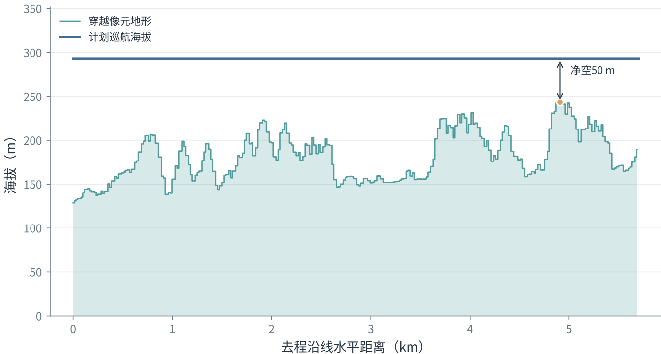
第一问：O01至S009沿线地形与净空
