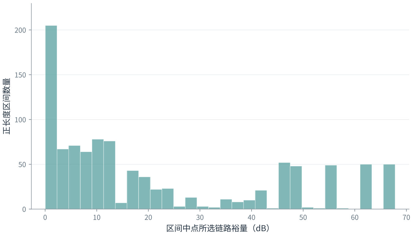
第三问：已分割区间中点链路裕量分布
