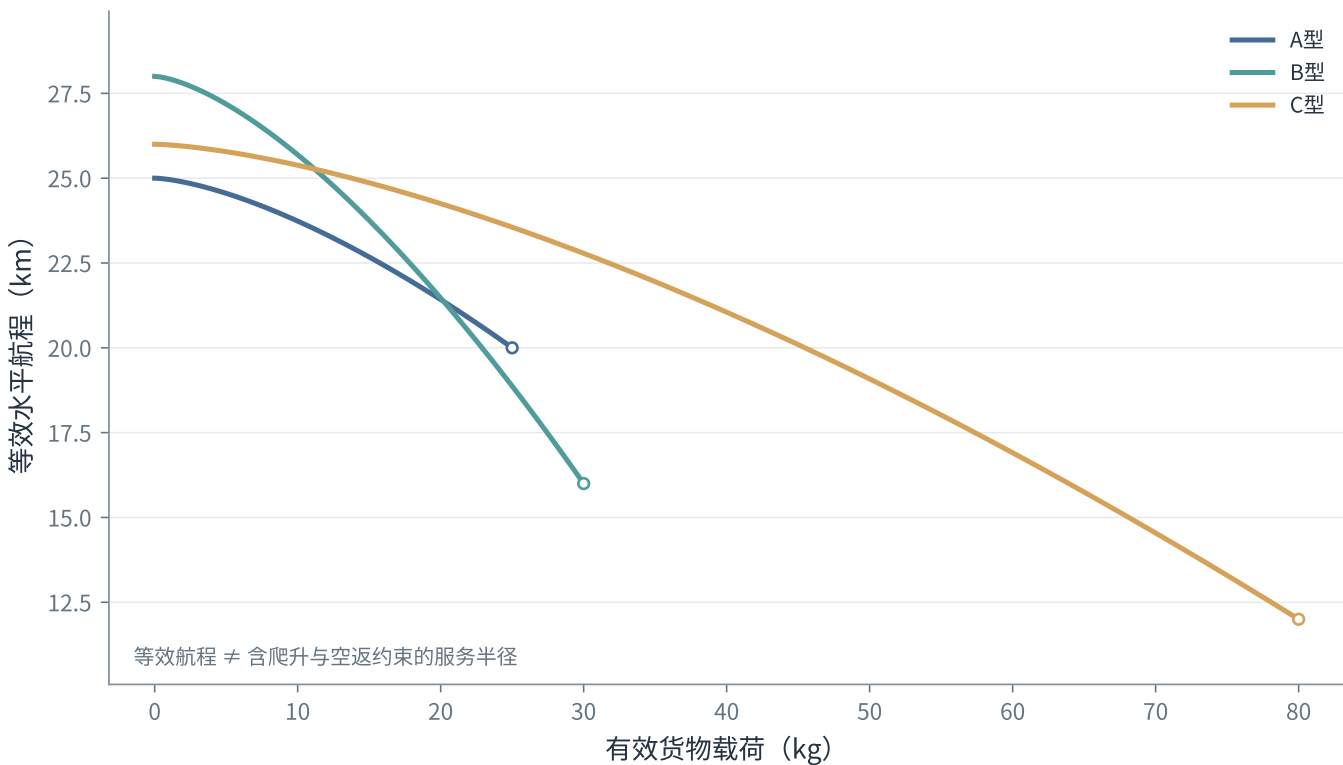
异构机型载荷—等效航程关系
