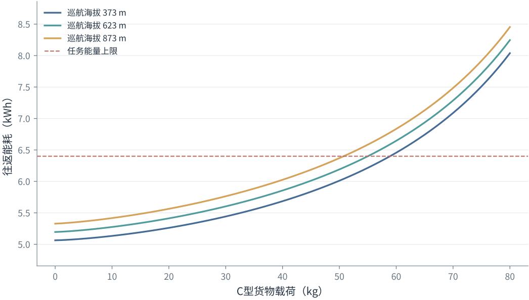
C 巡航海拔改变时的载荷—能耗截面
