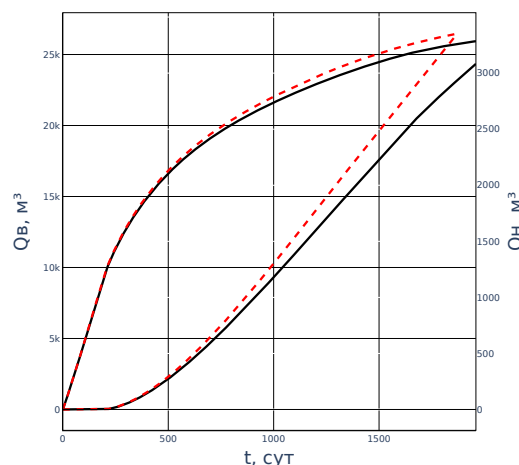
Рис. 2: Накопленные дебеты воды и нефти добывающей скважины
