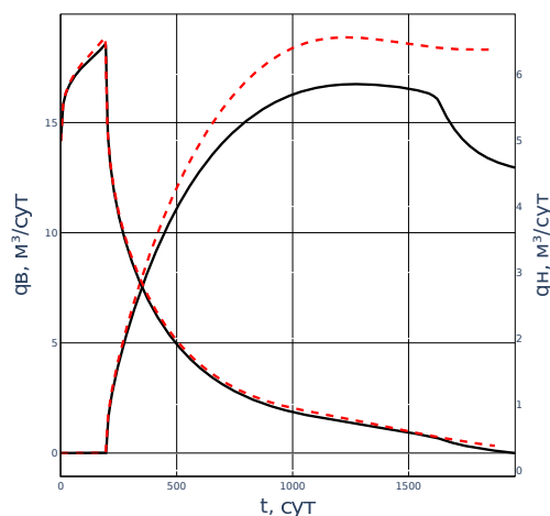
Рис. 1: Дебеты воды и нефти добывающей скважины
