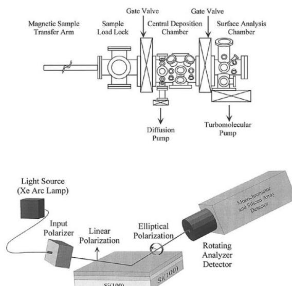
apparatus diagram:
