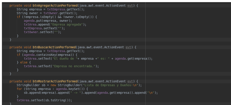
Figura 8: Método para agregar el nombre de la empresa y el dueño.
