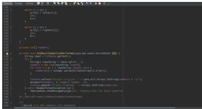
Figura 4: Código de la interfaz de Merge-Sort.
