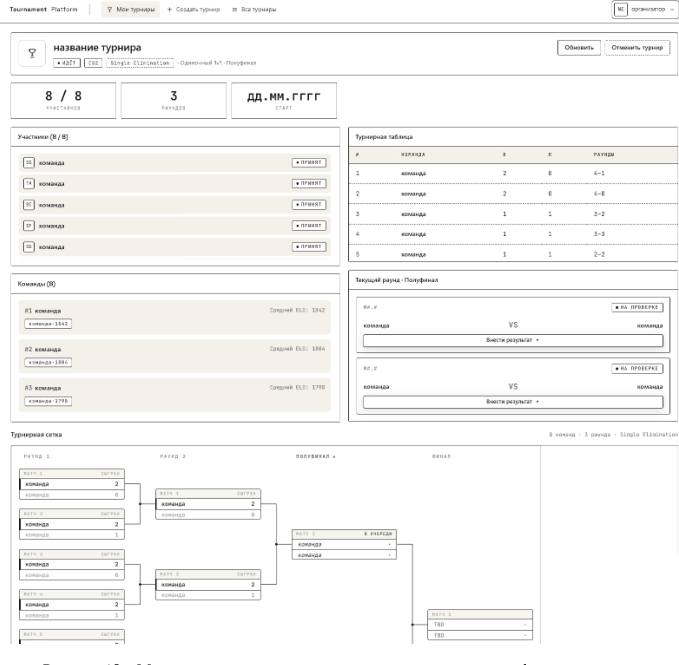
Рисунок 18 – Макет страницы запущенного турнира, проводимого в формате сетки
