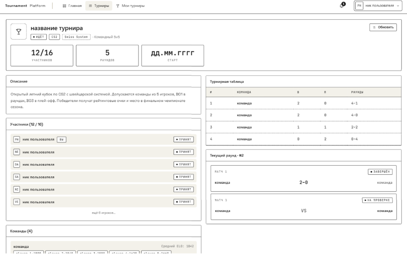
Рисунок 11 – Макет страницы запущенного турнира с швейцарской системой проведения
