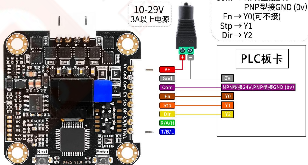
与PLC板卡连接示意图
