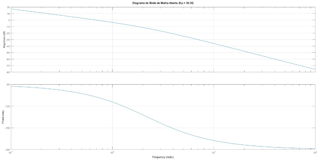
Figura 7: Diagrama de Bode de malha aberta ( L(s) ).
