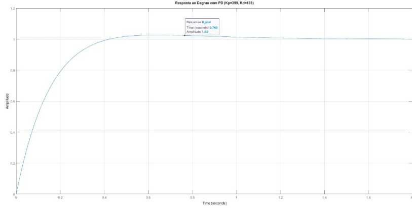
Figura 6: Resposta ao degrau com controlador PD ( T_s < 1s ).
