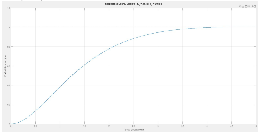
Figura 12: Resposta ao degrau do sistema em malha fechada com controlador proporcional e T_s = 0,015s .
