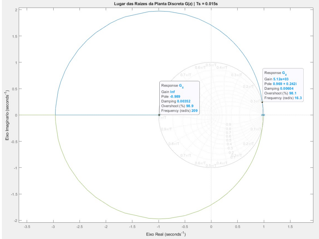
Figura 10: Lugar das Raízes da planta discreta G(z) com T_s = 0,015s .
