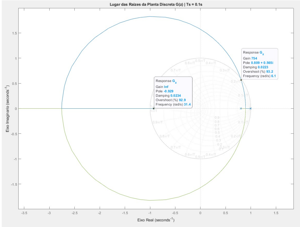
Figura 9: Lugar das Raízes da planta discreta G(z) .
