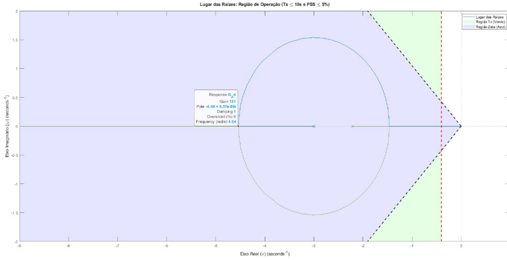
Figura 5: Lugar das Raízes com a introdução de um zero em s = -3 (Ação PD).
