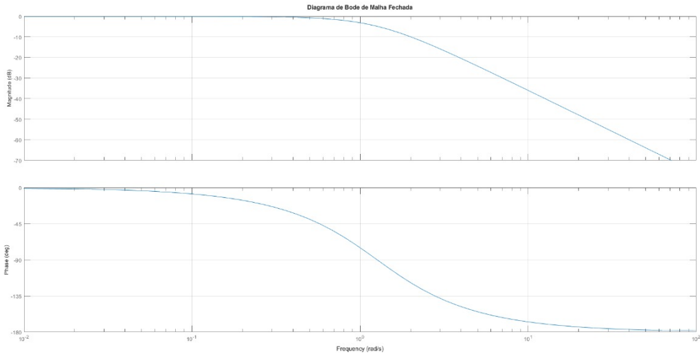
Figura 8: Diagrama de Bode de malha fechada ( H(s) ).
