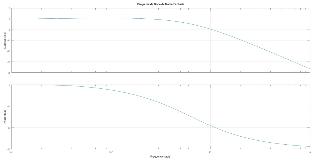
Figura 7: Diagrama de Bode de malha fechada H(s) : magnitude e fase.
