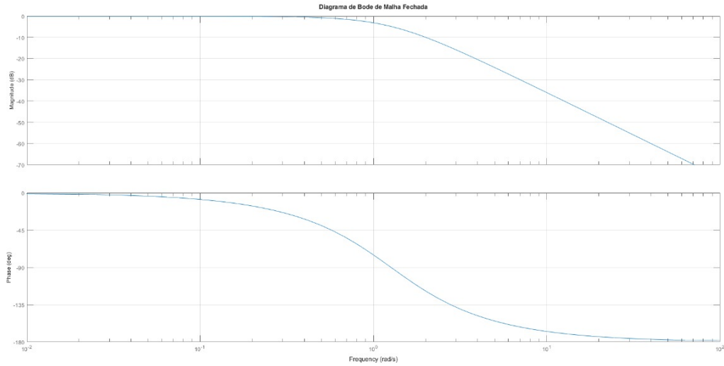
Figura 7: Diagrama de Bode de malha fechada ( H(s) ).
