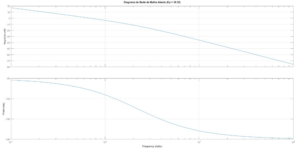
Figura 6: Diagrama de Bode de malha aberta ( L(s) ).
