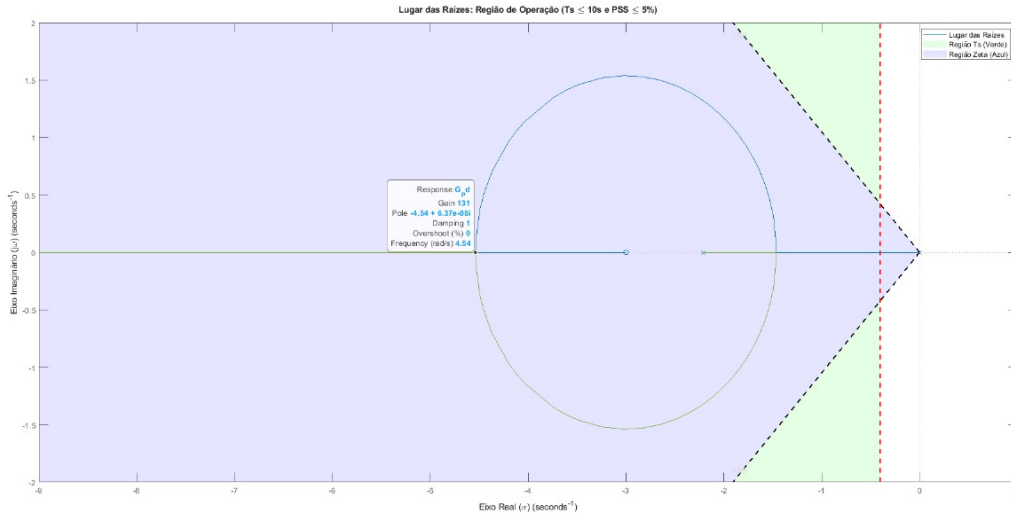
Figura 5: Alteração do Lugar das Raízes com a introdução de um zero em s = -3 (Ação PD).
