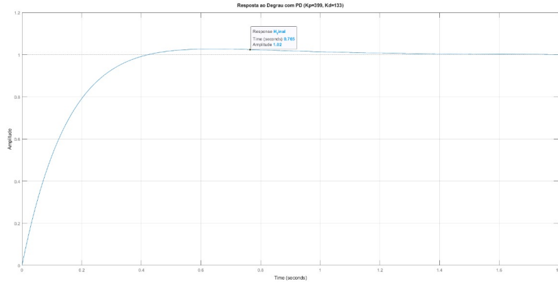
Figura 6: Resposta ao degrau com controlador PD sintonizado para alta velocidade ( T_s < 1s ).
