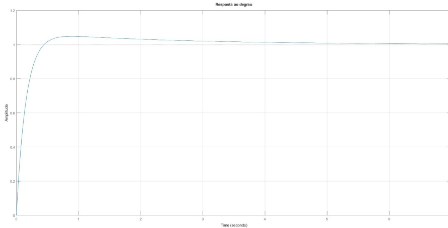
Figura 5: Resposta ao degrau com controlador PID.
