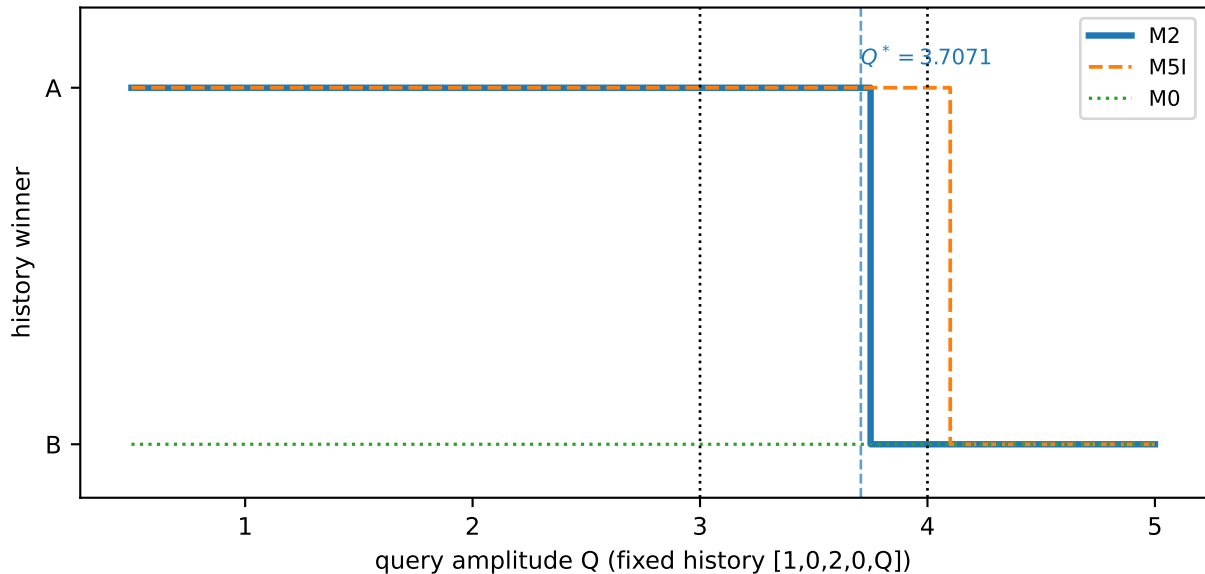
(d) The realized counterfactual flip (Sprint 4.2-B): margins +0.2587 \rightarrow -0.1559
