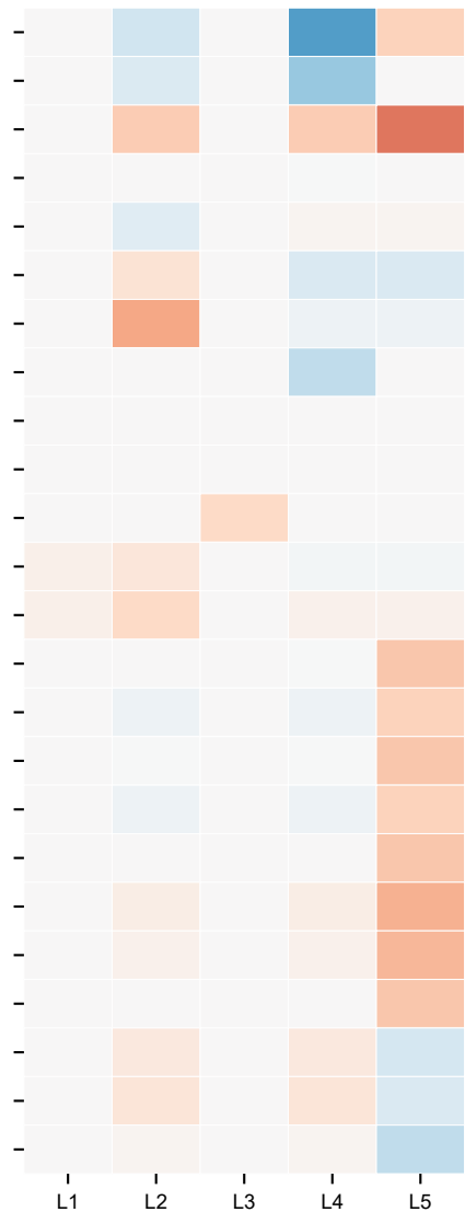
NoLSTM
