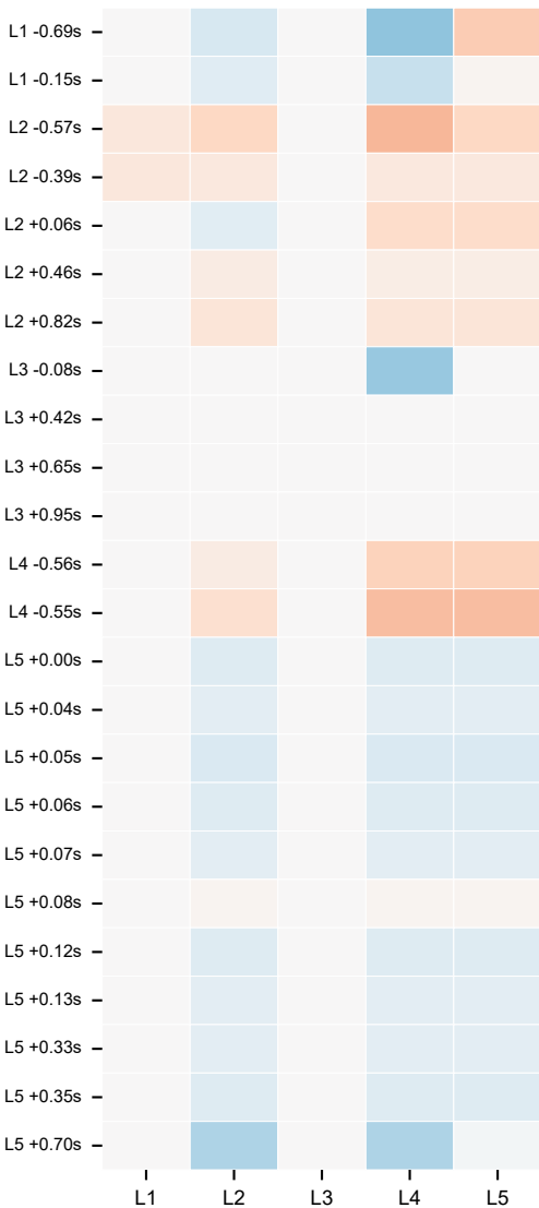
NoConv
