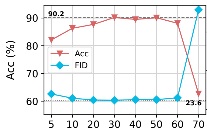
CelebA
